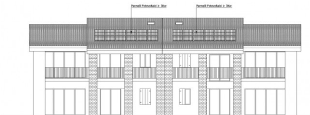
PROSPETTO OVEST
