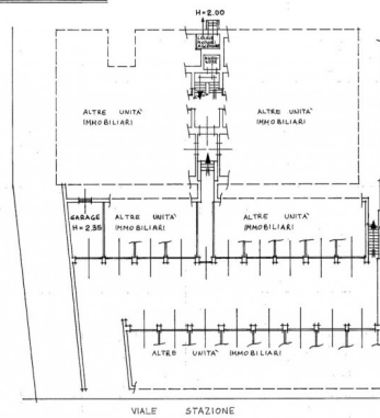
PIANTA PIANO INTERRATO
